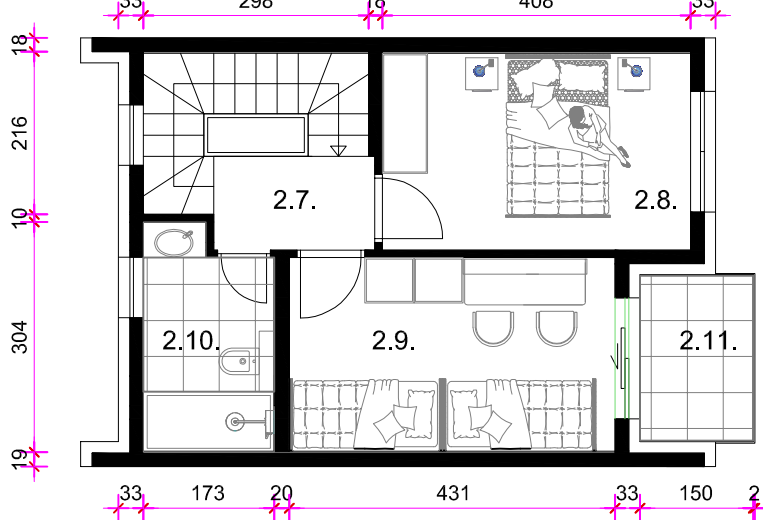
TLOCRT STANA 2 UVUČENI KAT
