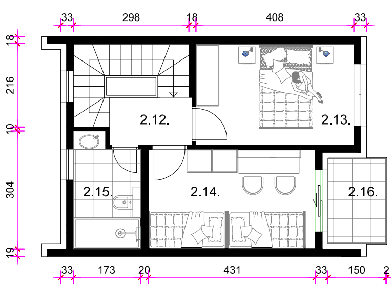
TLOCRT STANA 2 UVUČENI KAT
