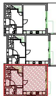
TLOCRT PRIZEMLJA
