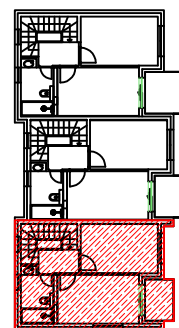
TLOCRT 1. KATA
