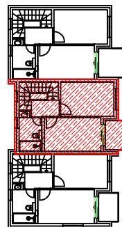
TLOCRT 1. KATA
