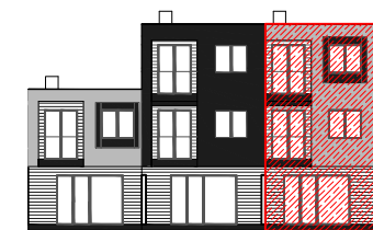
JUGOISTOČNO DS1 MJ 1:100
