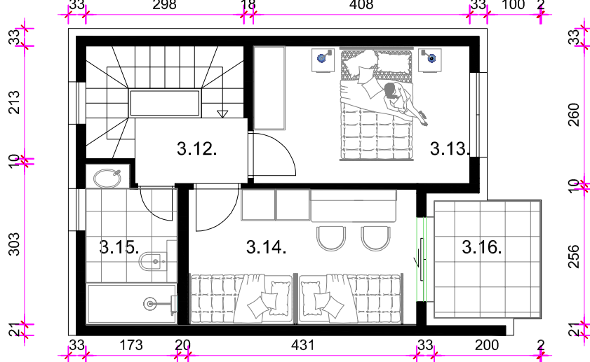
TLOCRT STANA 3 UVUČENI KAT
