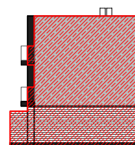
SJEVEROISTOČNO DS1 MJ 1:100
