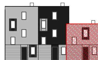
SJEVEROZAPADNO DS1 MJ 1:100
