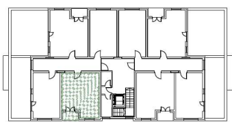
TLOCRT UVUČENOG KATA
