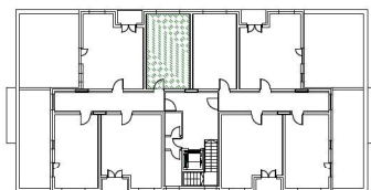
TLOCRT UVUČENOG KATA
