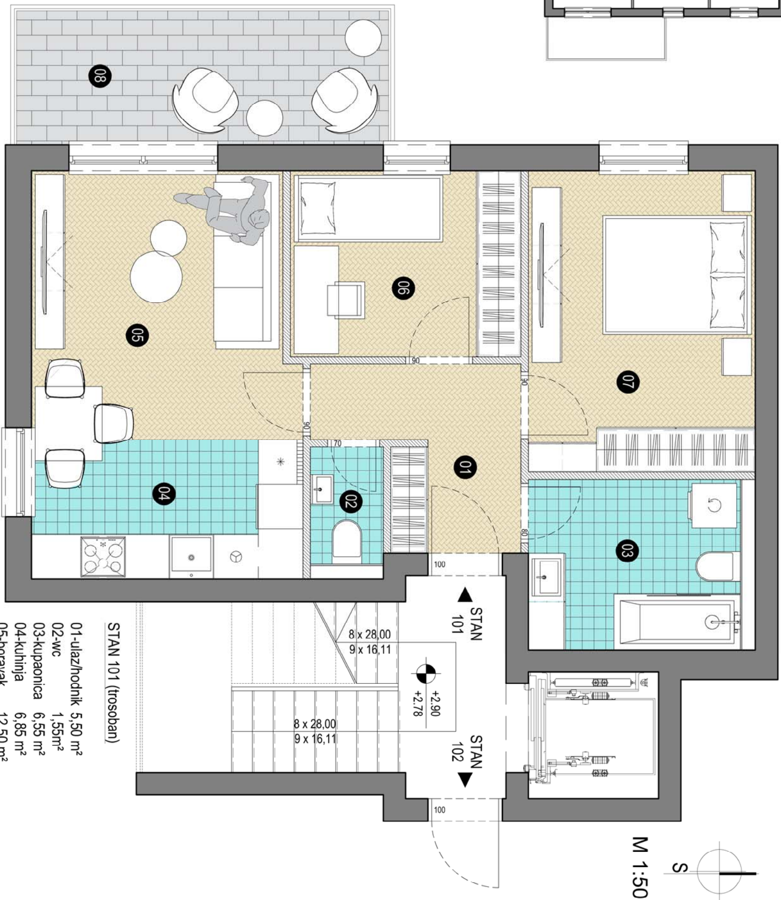
STAN 101 PRIKAZ POKRŠINA PROSTORIJA I UKUPNA POKRŠINA STANA
