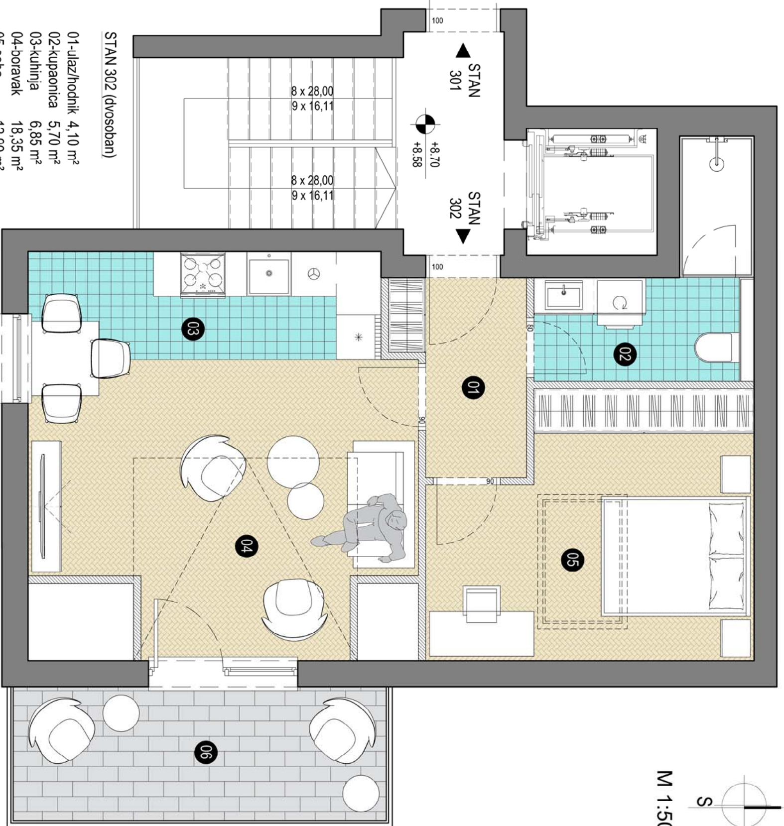
STAN 302 PRIKAZ POKRŠINA PROSTORIJA I UKUPNA POKRŠINA STANA
