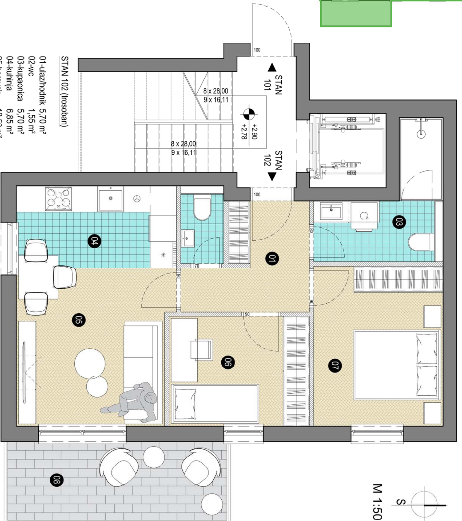
STAN 102 PRIKAZ POKRIVNOSTI PROSTORIJA I UKUPNA POKRIVNOSTI STANA
