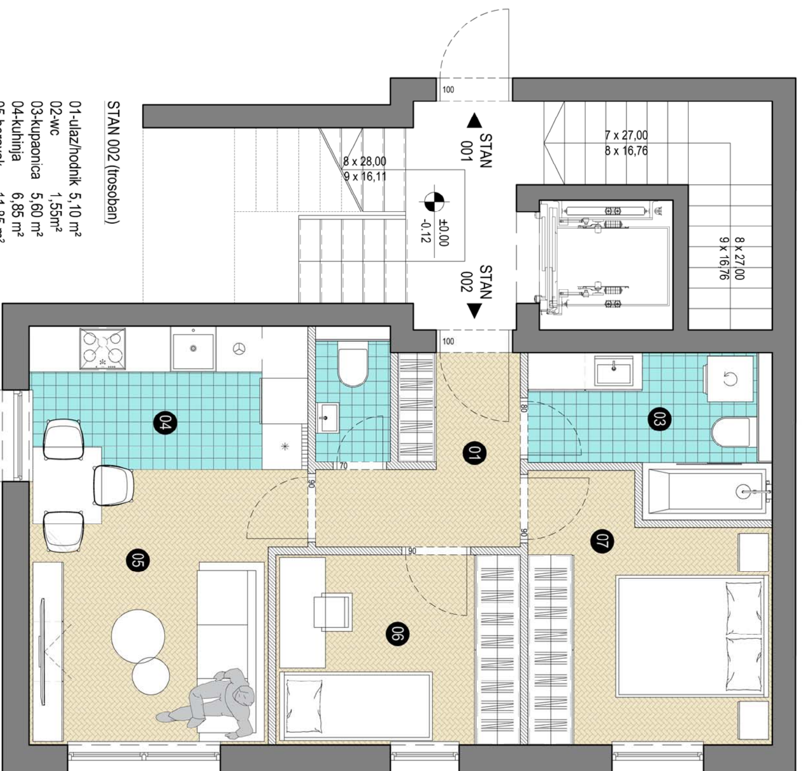
STAN 002 PRIKAZ POKRIVNOSTI PROSTORIJA I UKUPNA POKRIVNOSTI STANA
