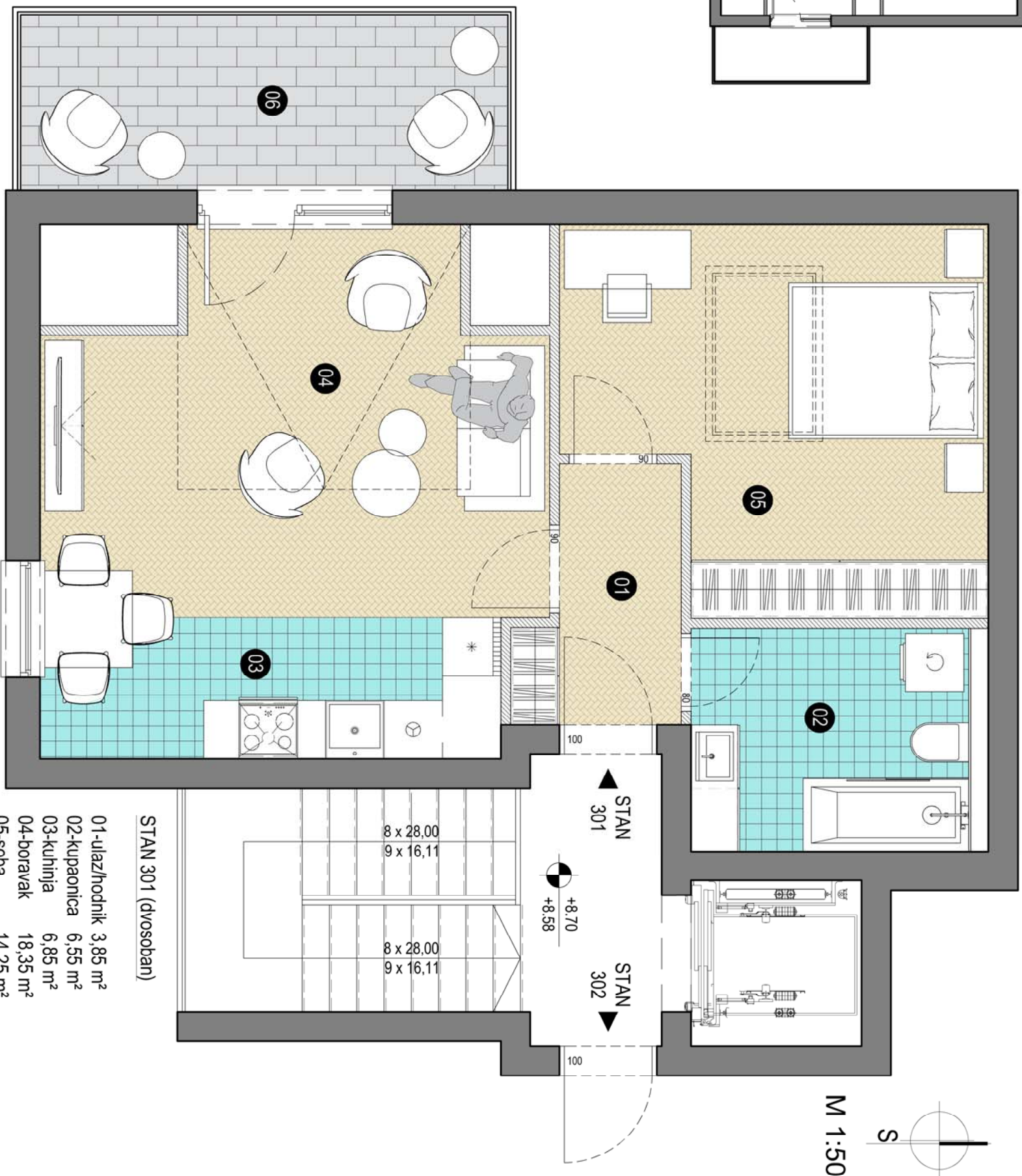
STAN 301 PRIKAZ POKRŠINA PROSTORIJA I UKUPNA POKRŠINA STANA
