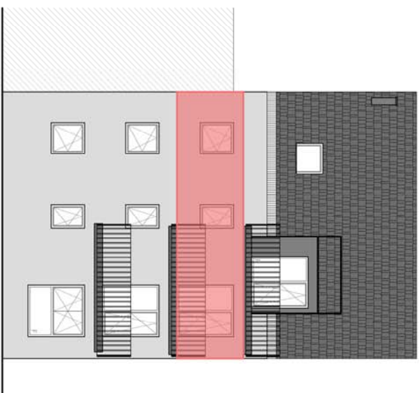
PRIKAZ STANA NA ZAPADNOM PROČELJU
