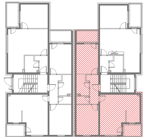
TLOCRT KATA
