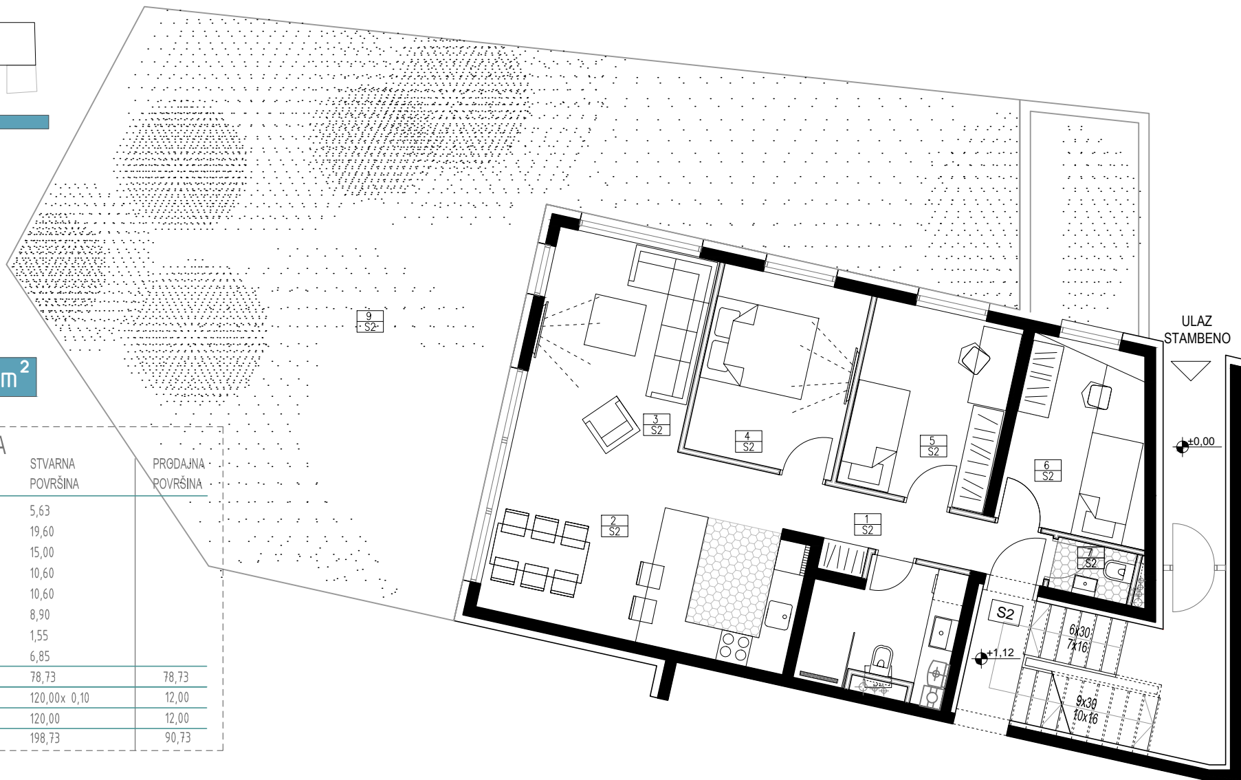
shema prizemlja
