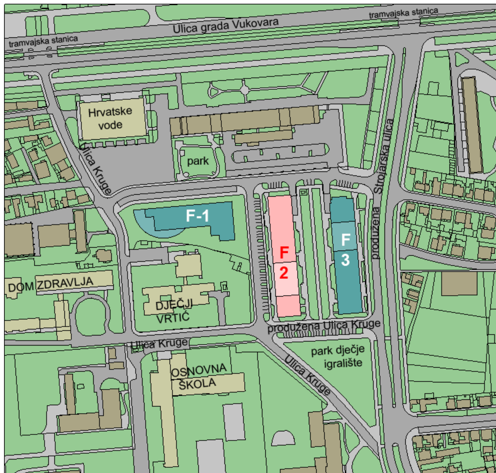
STAMBENO POSLOVNA GRAĐEVINA RADNOG NAZIVA F2 U NASELJU KRUGE-SITUACIJA
